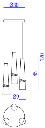
FUENTE 3 230V AC LED max 3x6W E14 CE IP20
