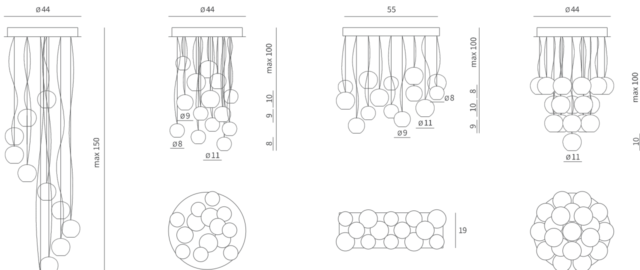
AIRE 14X 14x20W G4 12V + \ominus - AIRE 14XP 14x20W G4 12V + \ominus - AIRE 21D 21x20W G4 12V + \ominus - CE IP20
