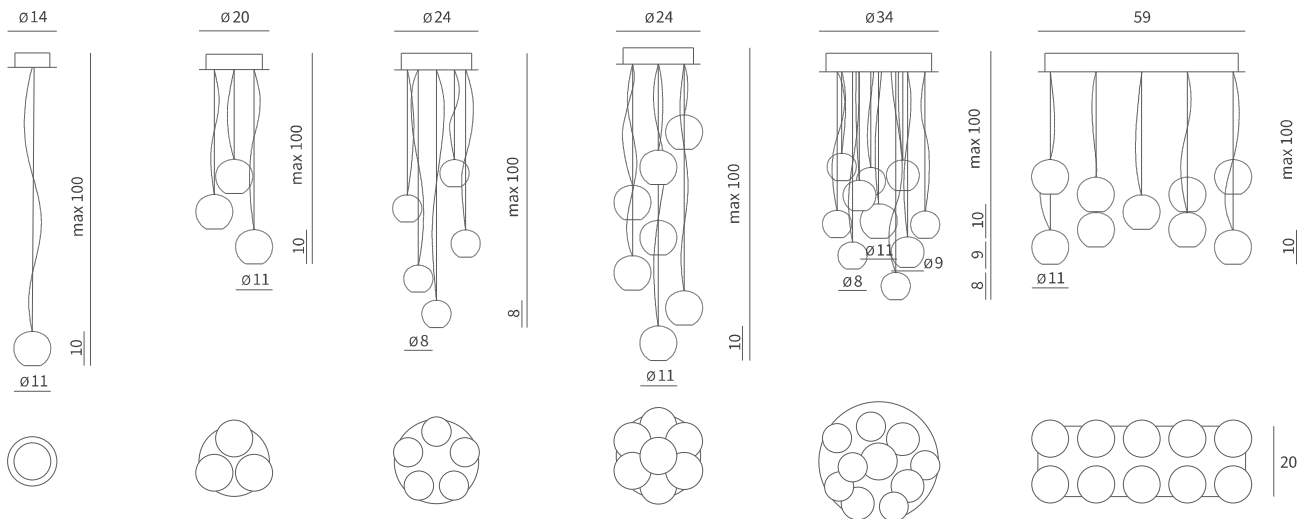
AIRE 1D 1x20W G4 12V + \ominus - AIRE 3D 3x20W G4 12V + \ominus - AIRE 5M 5x20W G4 12V + \ominus - AIRE 7D 7x20W G4 12V + \ominus - AIRE 10X 10x20W G4 12V + \ominus - AIRE 10DP 10x20W G4 12V + \ominus - CE IP20
